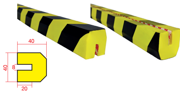
Model : BJSP-6 Dimension : 4 x 4 x 100
