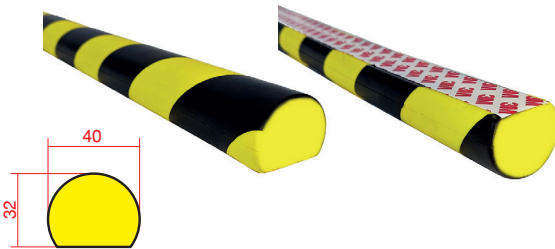
Model : BJSP-5 Dimension : 4 x 3.2 x 100
