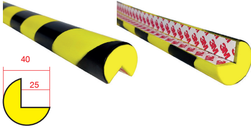
Model : BJSP-1 Dimension : 4 x 4 x 100
