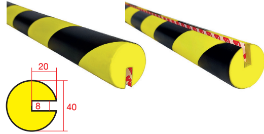
Model : BJSP-2 Dimension : 4 x 4 x 100
